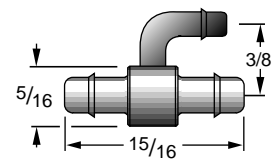
RT4-3L-4 S/S
