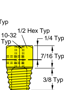
1/8LT-10F
